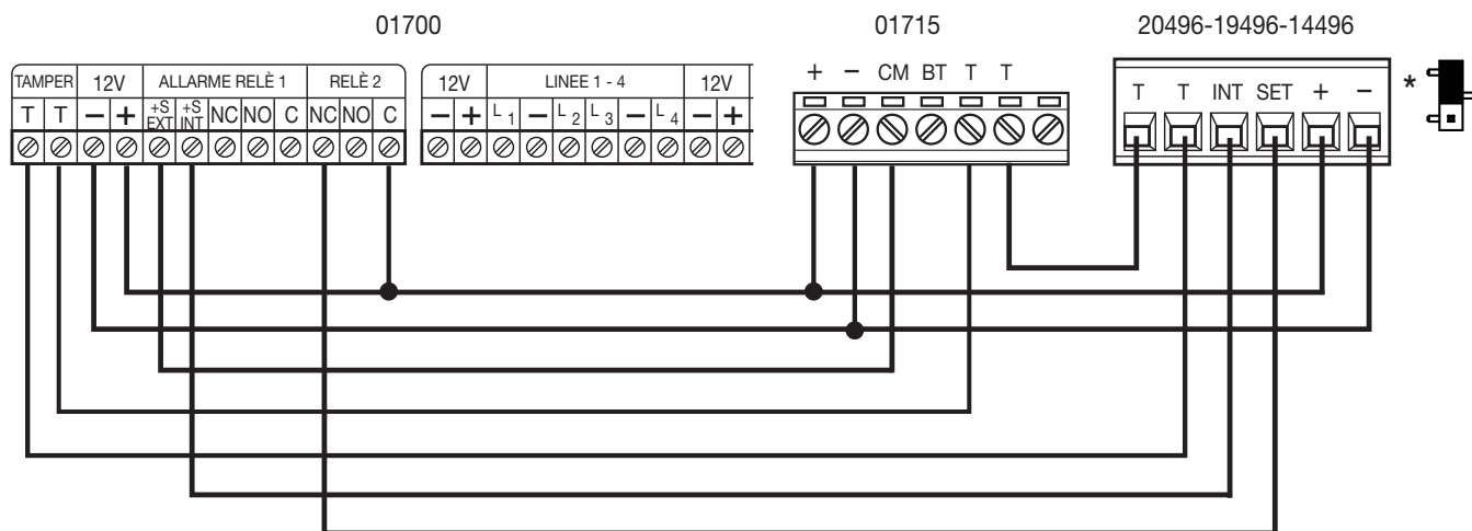
ESEMPIO DI COLLEGAMENTO DELLA CENTRALE CON LA SIRENA DA ESTERNO 01715 E LA SIRENA DA INTERNO 20496-19496-14496
