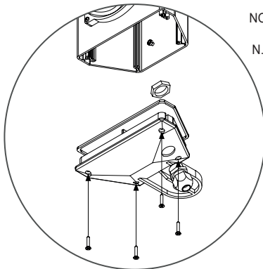
MONTAGGIO COPERCHIO SU SEMAFORO COVER ASSEMBLY ON TRAFFIC LIGHTS
