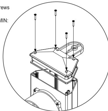
MONTAGGIO COPERCHIO SU SEMAFORO COVER ASSEMBLY ON TRAFFIC LIGHTS
