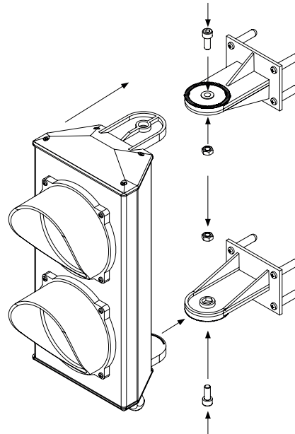
FISSAGGIO CORPO SU STAFFA BODY FIXING ON BRACKET
